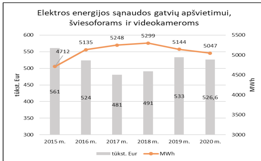
2 pav. Elektros energijos sąnaudų Šiaulių miesto gatvių apšvietimui ir šviesoforams dinamika 2015 – 2020 m.
